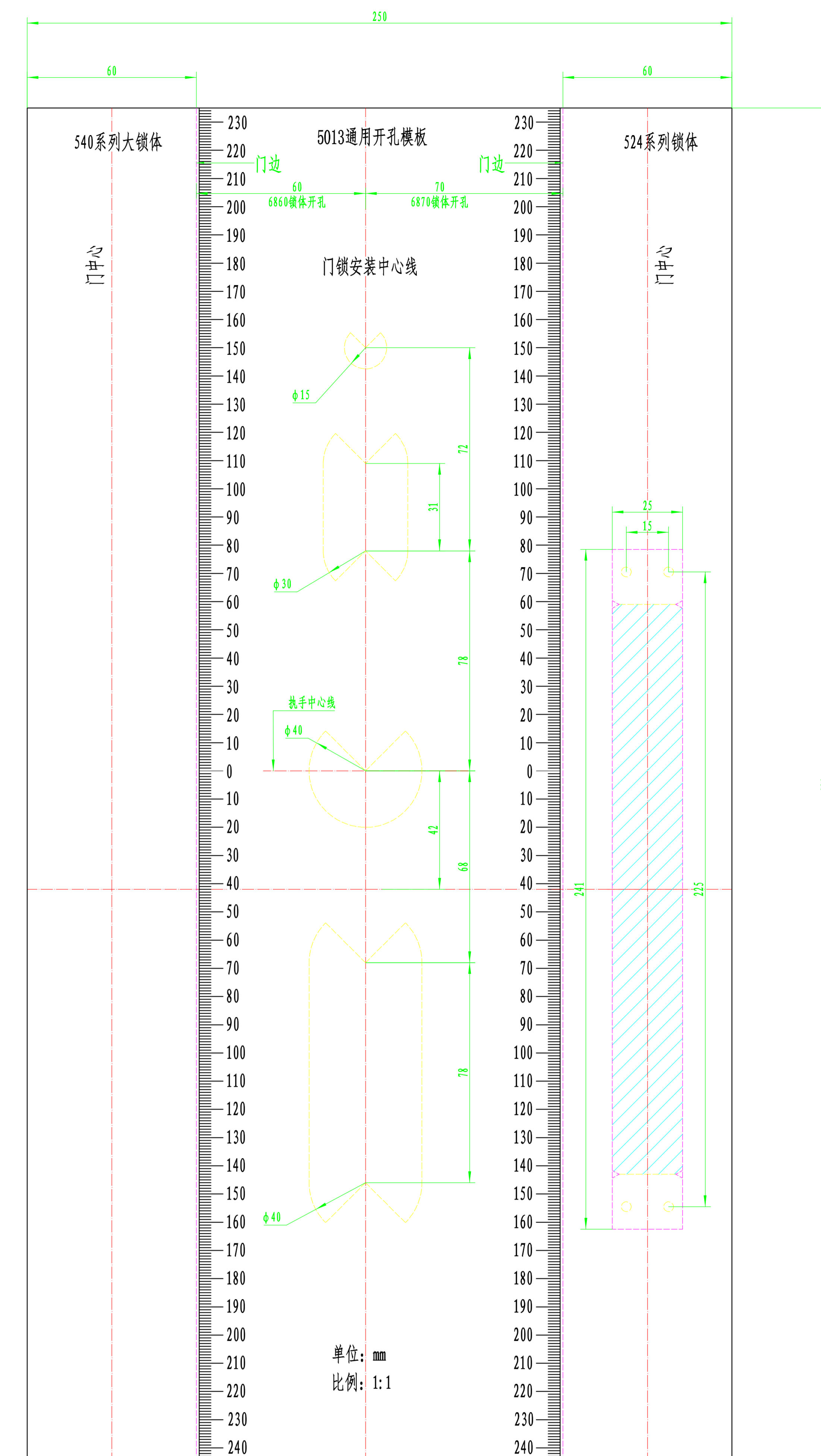
外形尺寸图
